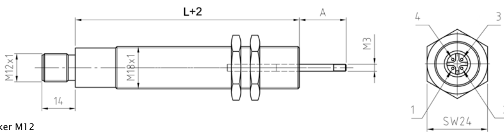
Anschluss: Stecker M12 Connection: Plug M12
